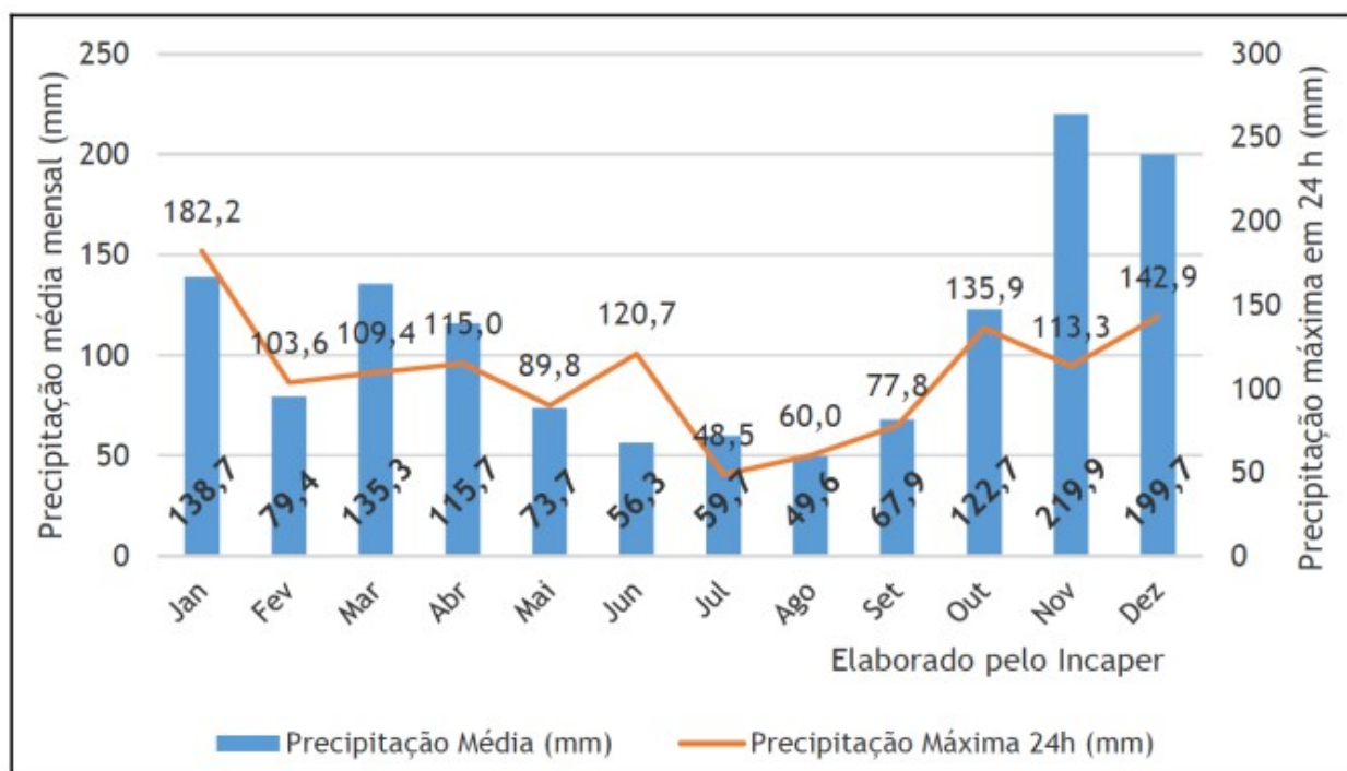
Figura 9: Média mensal de precipitação e valores máximos de precipitação acumulada em 24 horas, na região de Vila Velha - ES. Fonte de dados: INMET 15 - Normais Climatológicas do Brasil (1981 – 2010) e gráfico elaborado pelo Incaper 16 .
