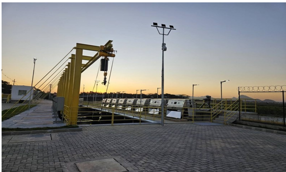
Foto 13: Estação de Bombeamento de Águas Pluviais Laranja. Crédito: Comunicação/SEDURB.
