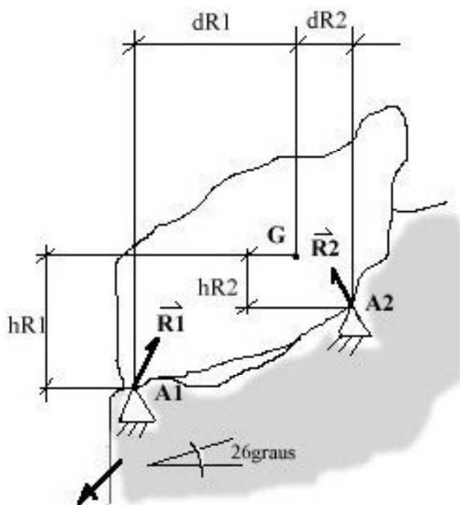
(b) Modelo geomecânico segundo o mecanismo de ruptura dos pontos de apoio do bloco rochoso
