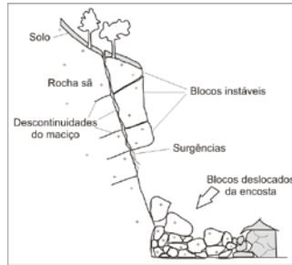
Figura 3.15 – Perfil esquemático do processo de queda de blocos.
