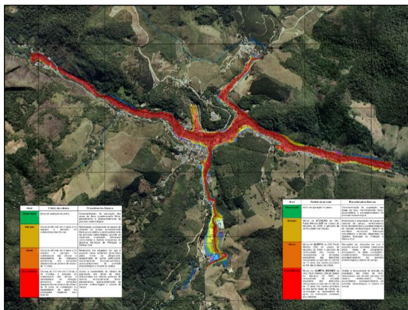
Figura 12: Áreas com risco de inundação na área urbana de Santa Leopoldina/ES. Fonte: Plano Diretor de Águas Pluviais (PDAP) do município.
