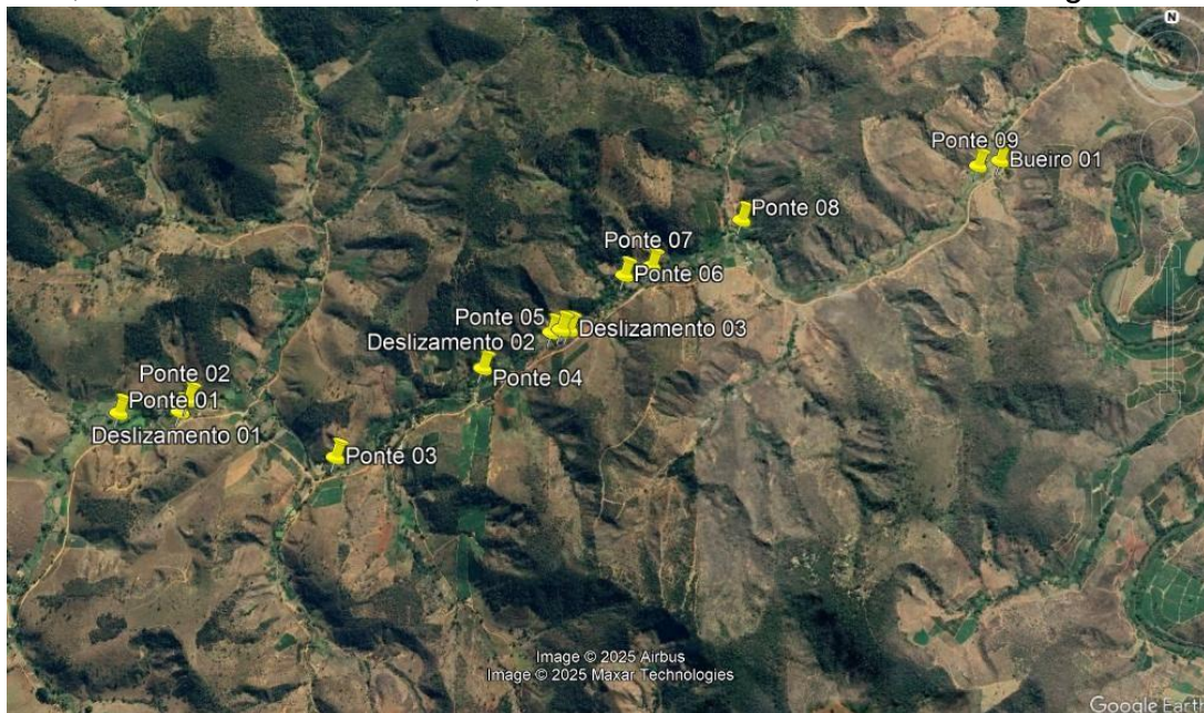
Pontes, bueiros e deslizamentos, ocorridos no trecho de estrada córrego criciúma.
