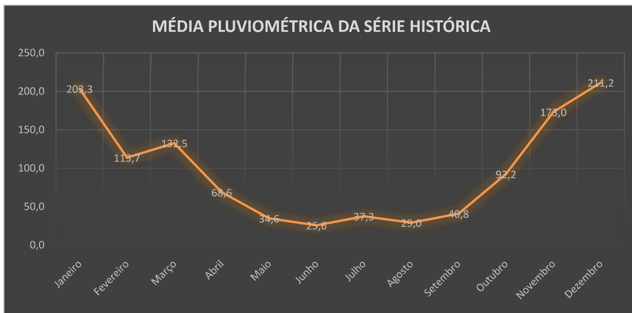
FIGURA 01. Gráfico 01. Média pluviométrica anual analisada entre 1958 a 2017 em mm/mês
